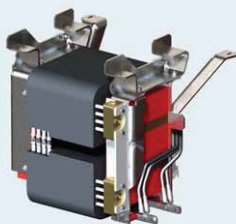
Wassergekühlte Filterdrossel 210 kW mit geschlossenem Wicklungsverguss
