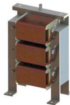
Schweißtransformator 60 kVA Welding transformer 60 kVA
